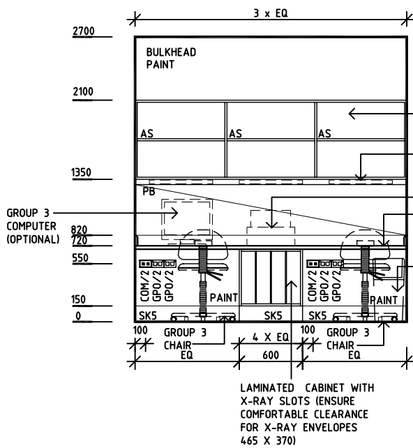
ELEVATION 1
