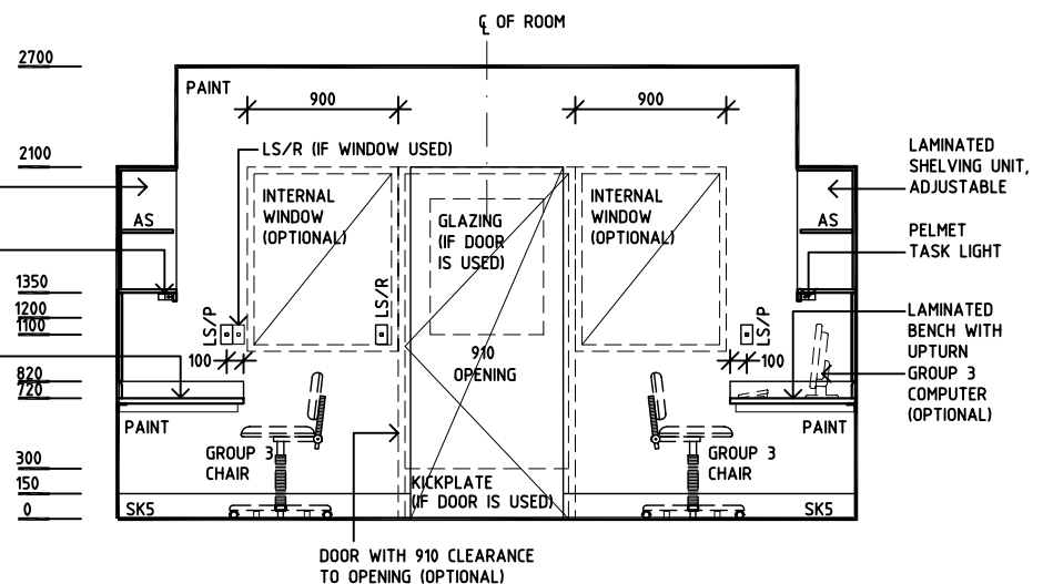
ELEVATION 2
