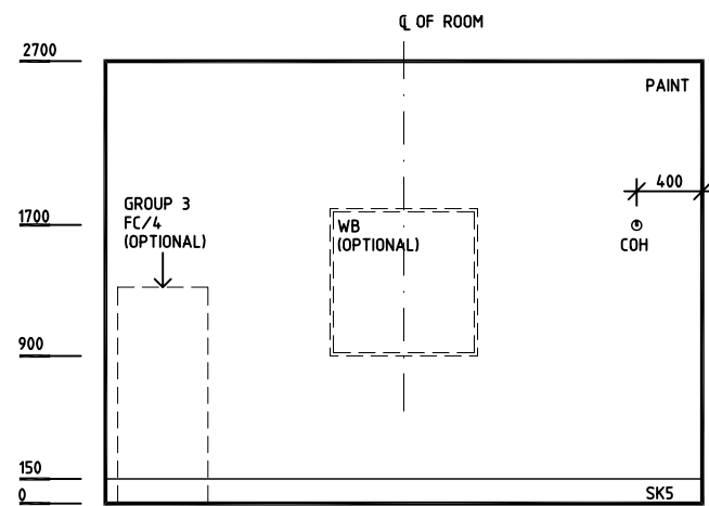
ELEVATION 2
