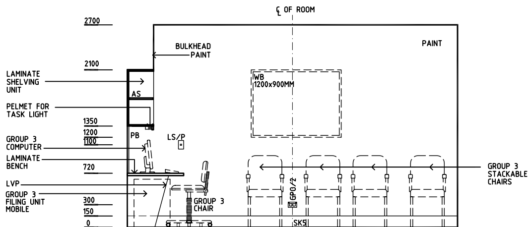
ELEVATION 4
