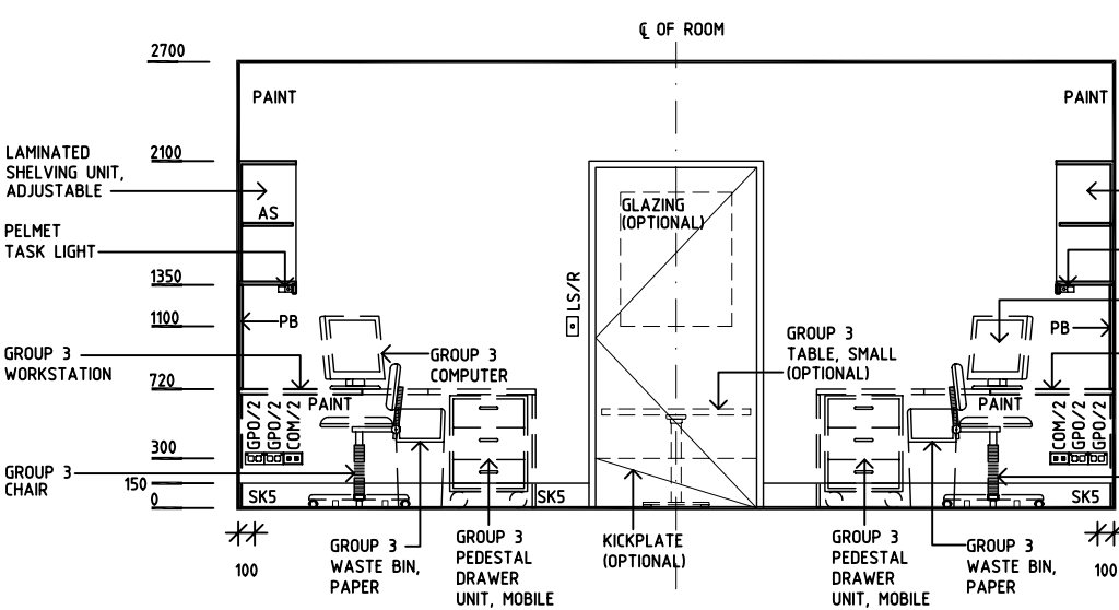
ELEVATION 3
