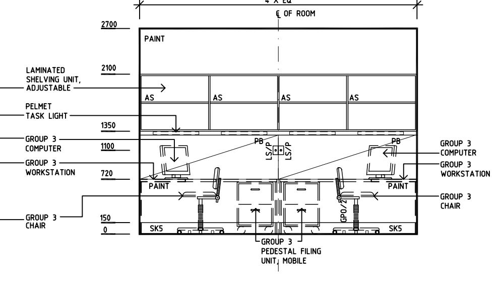
ELEVATION 4
