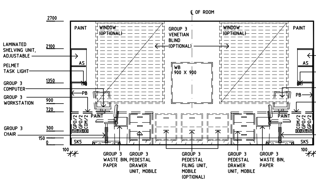
ELEVATION 1
