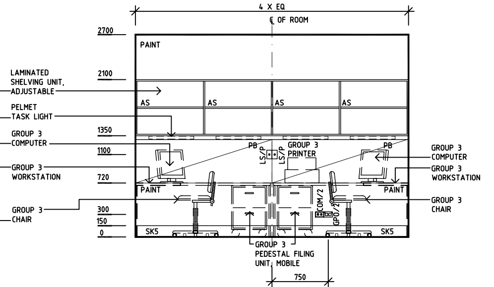
ELEVATION 2
