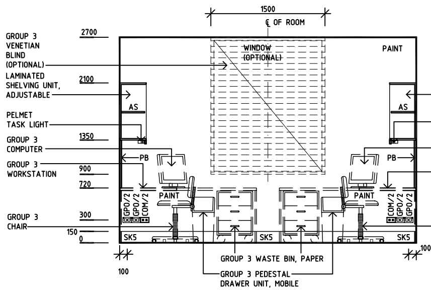
ELEVATION 1
