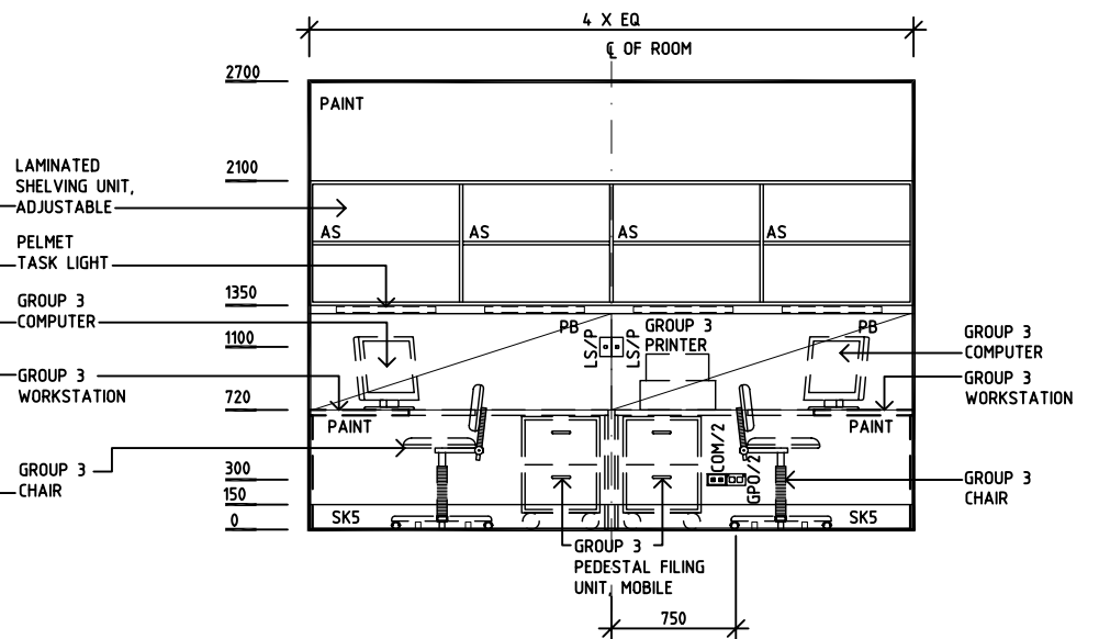
ELEVATION 2
