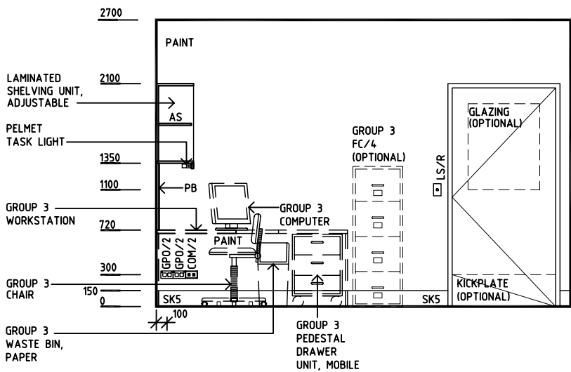
ELEVATION 3
