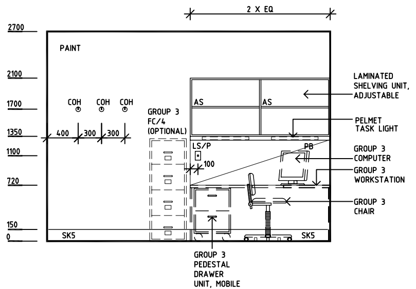
ELEVATION 4
