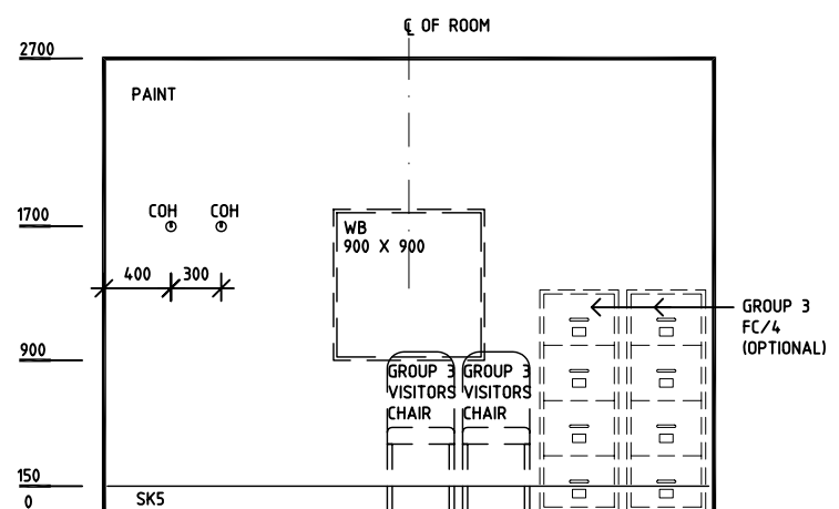
ELEVATION 2
