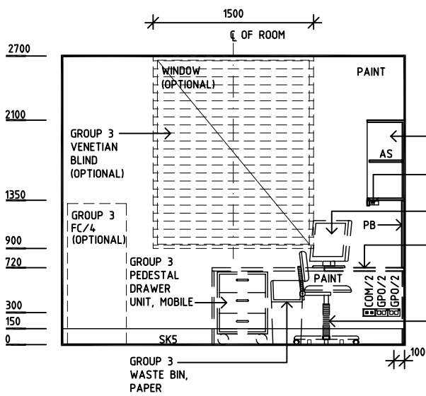
ELEVATION 1
