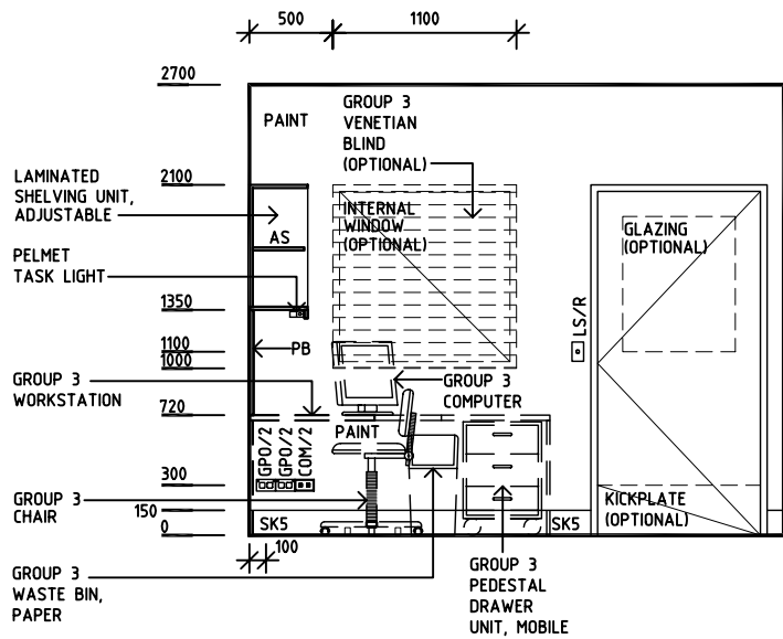
ELEVATION 3
