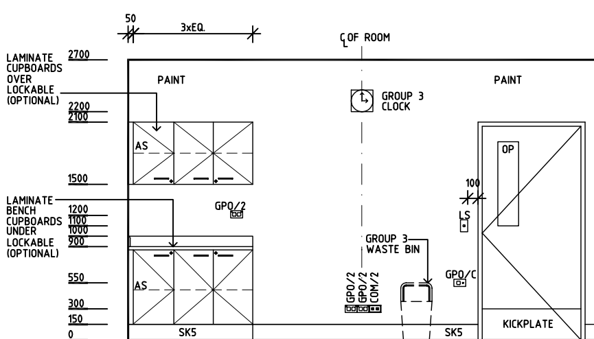
ELEVATION 3
