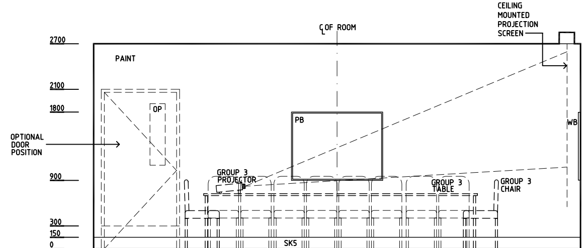
ELEVATION 4
