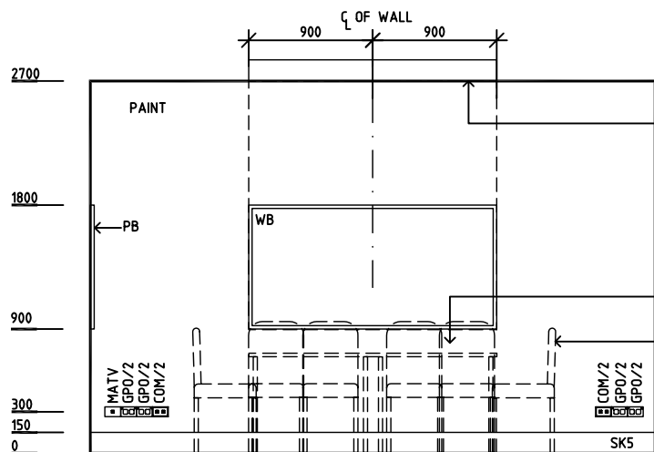
ELEVATION 1
