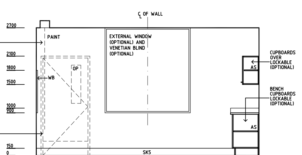
ELEVATION 2
