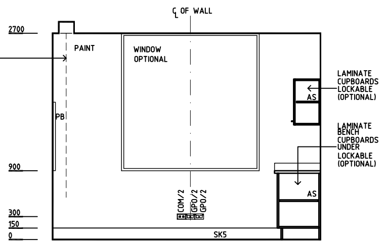
ELEVATION 2
