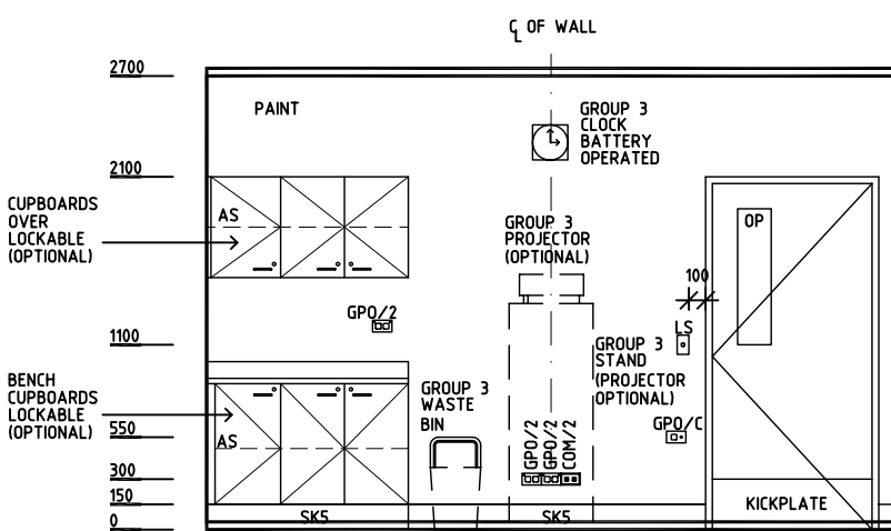
ELEVATION 3
