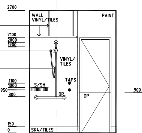
ELEVATION 4
