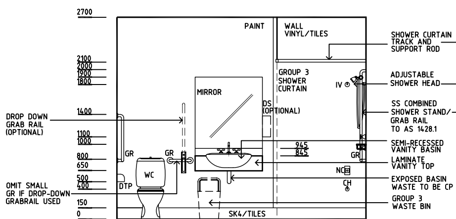
ELEVATION 3
