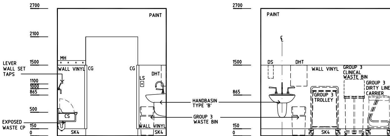
ELEVATION 3
