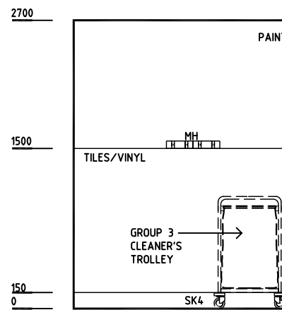
ELEVATION 4
