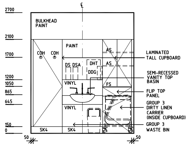
ELEVATION 4
