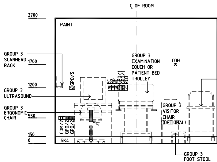
ELEVATION 1
