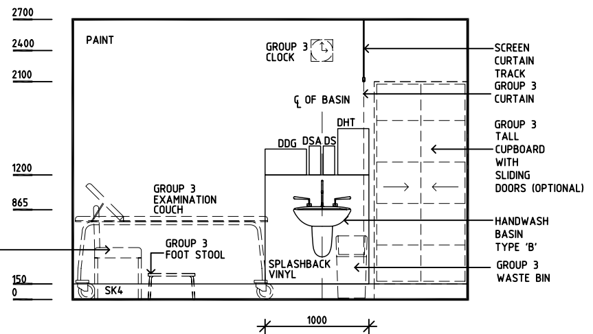
ELEVATION 2
