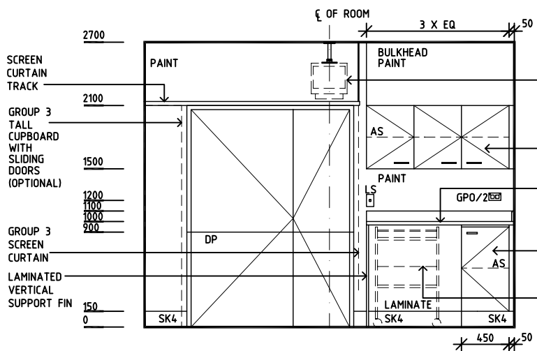
ELEVATION 3
