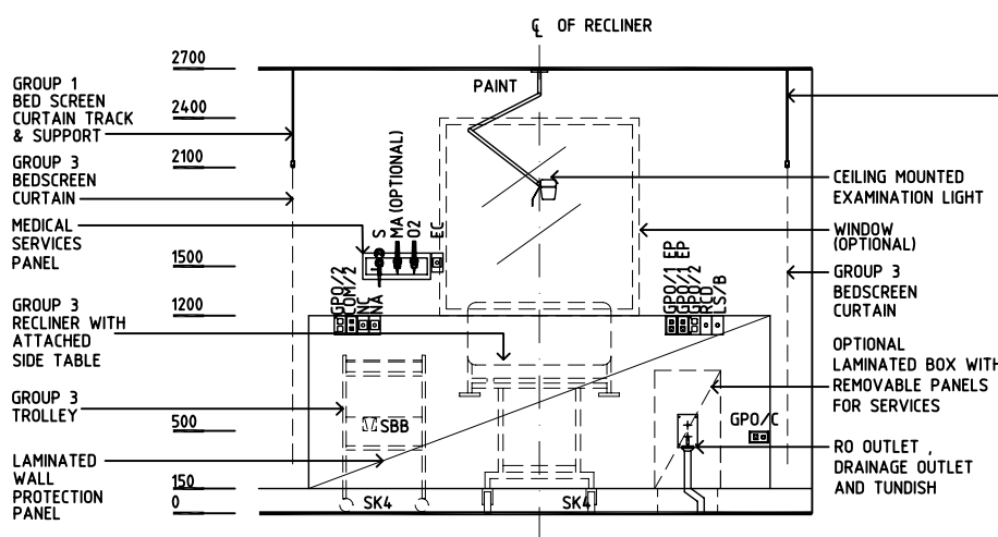
ELEVATION 1
