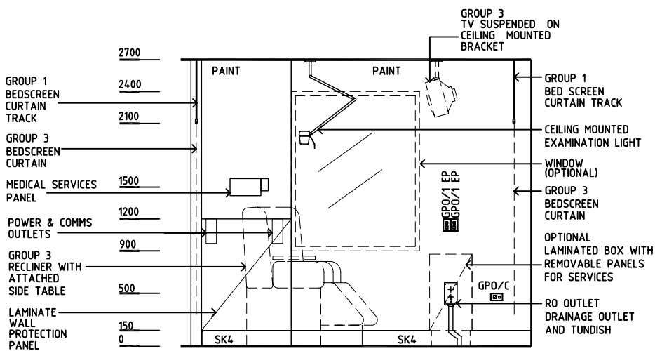
ELEVATION 1
