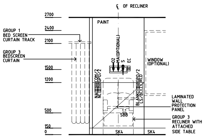
ELEVATION 3
