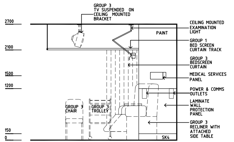
ELEVATION 2
