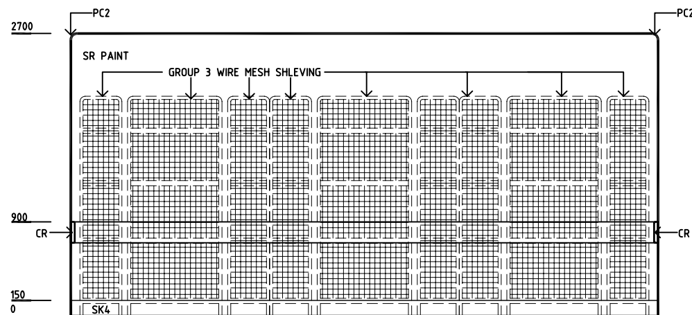
ELEVATION 4
