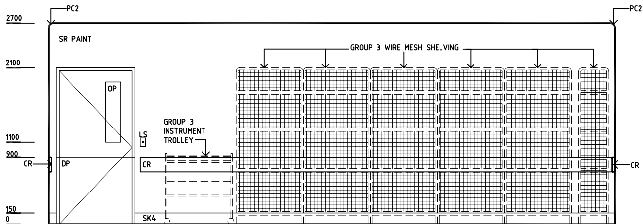
ELEVATION 3
