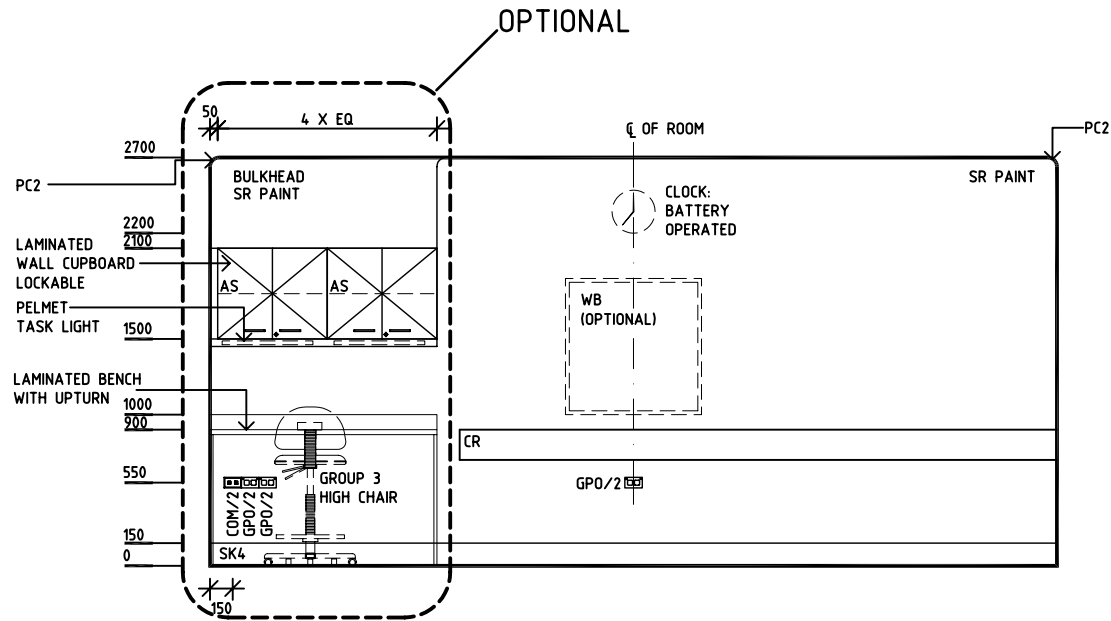
ELEVATION 2
