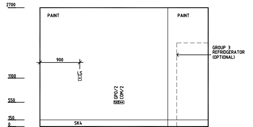
ELEVATION 2
