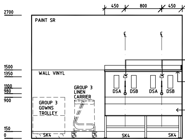
ELEVATION 1
