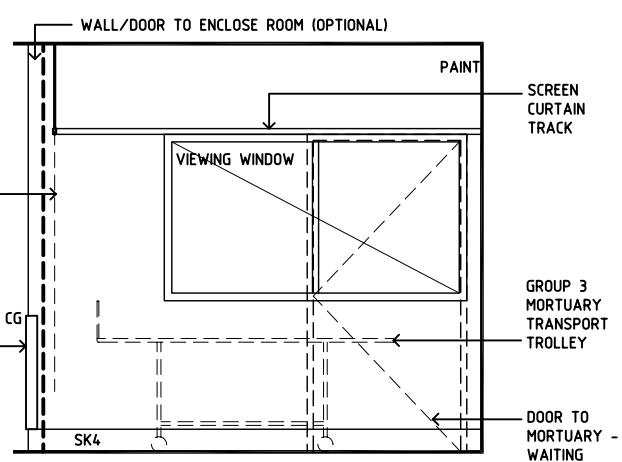
ELEVATION 4
