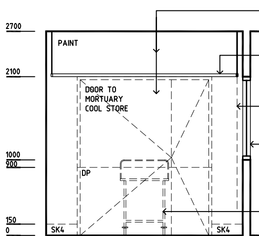
ELEVATION 3
