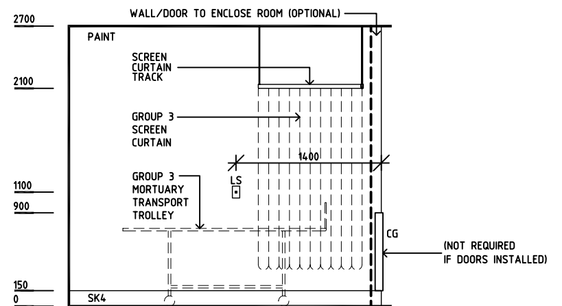
ELEVATION 2
