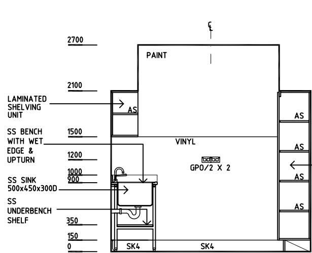
ELEVATION 1
