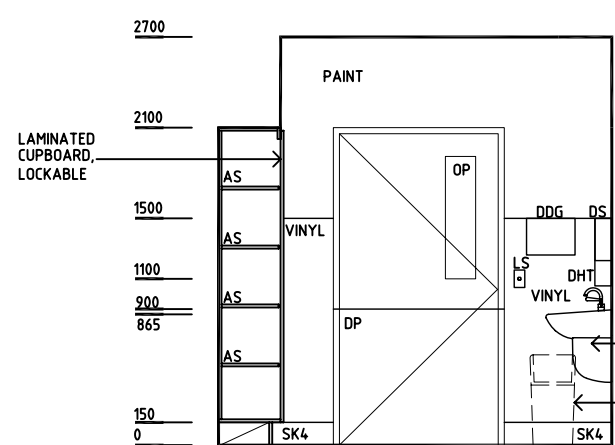
ELEVATION 3
