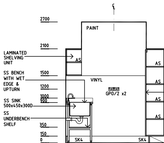
ELEVATION 1
