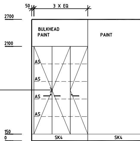
ELEVATION 2
