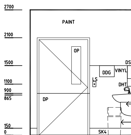
ELEVATION 3
