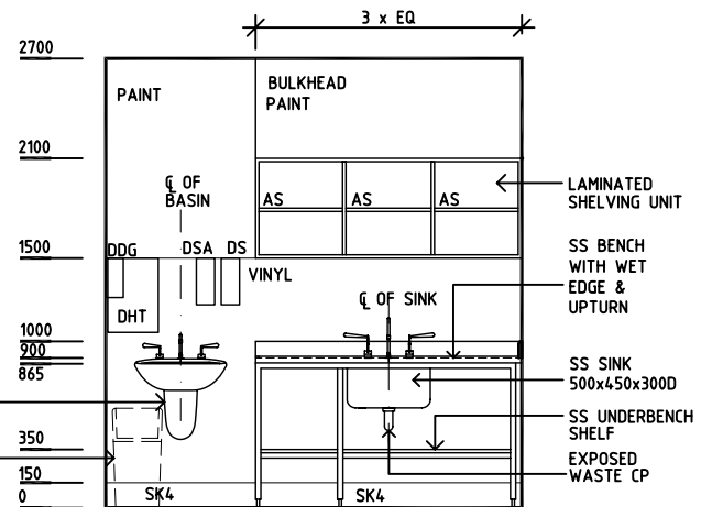
ELEVATION 4
