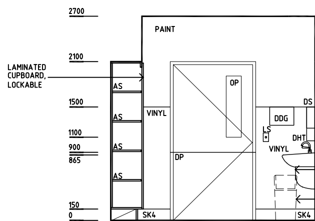
ELEVATION 3
