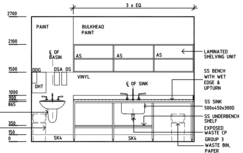
ELEVATION 4
