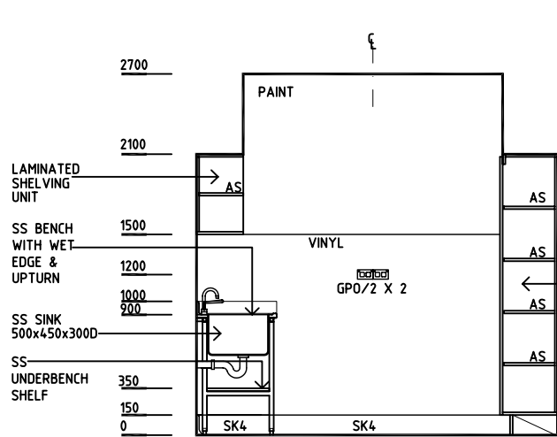
ELEVATION 1
