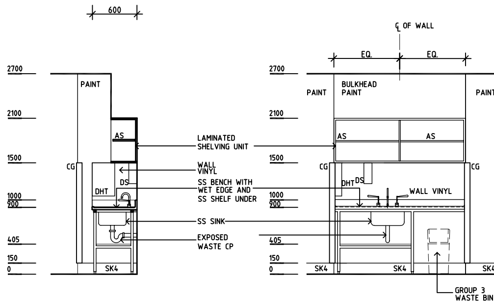
ELEVATION 1
