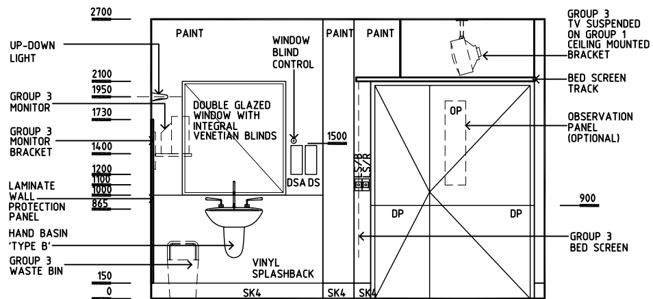
ELEVATION 3
