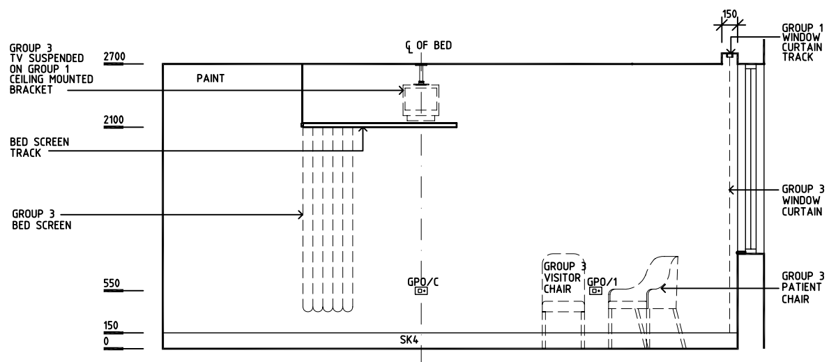
ELEVATION 4
