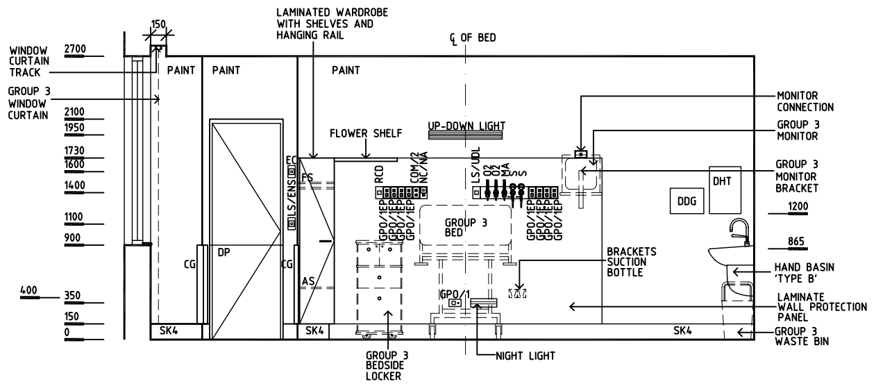
ELEVATION 2
