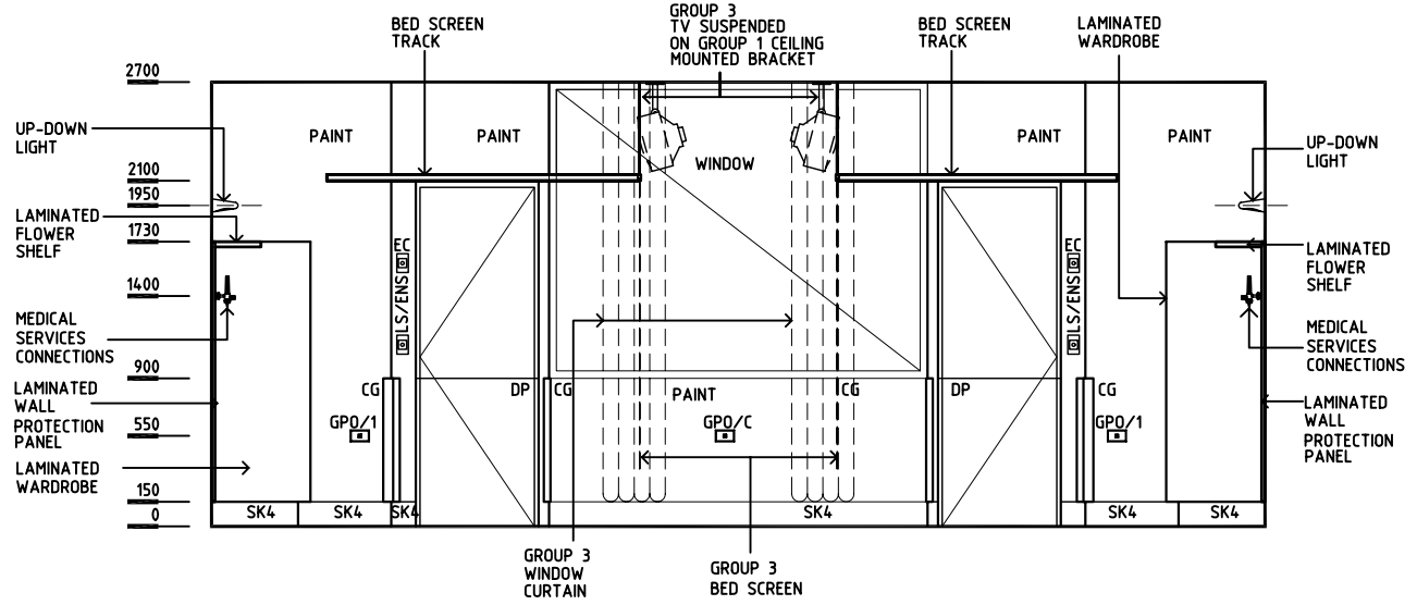
ELEVATION 1
