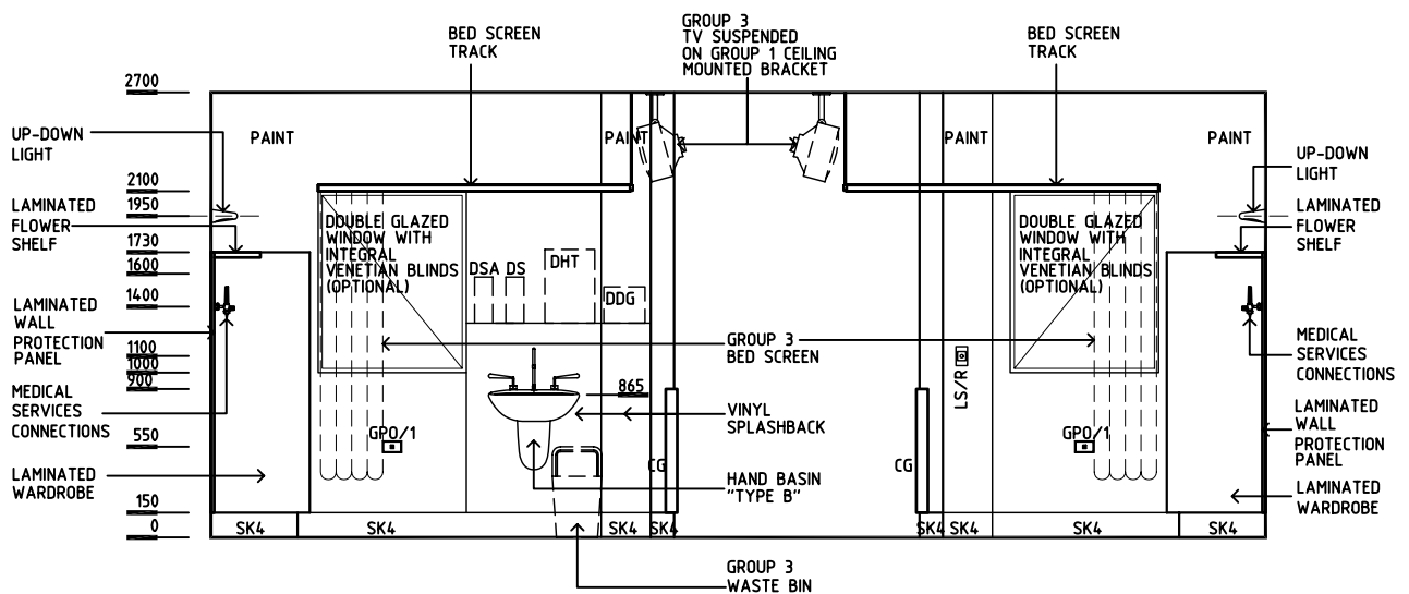
ELEVATION 3
