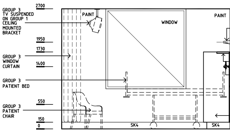
ELEVATION 1
