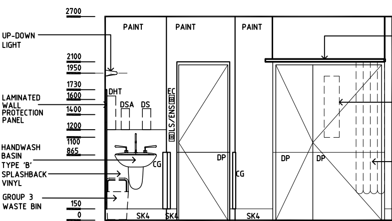
ELEVATION 3
