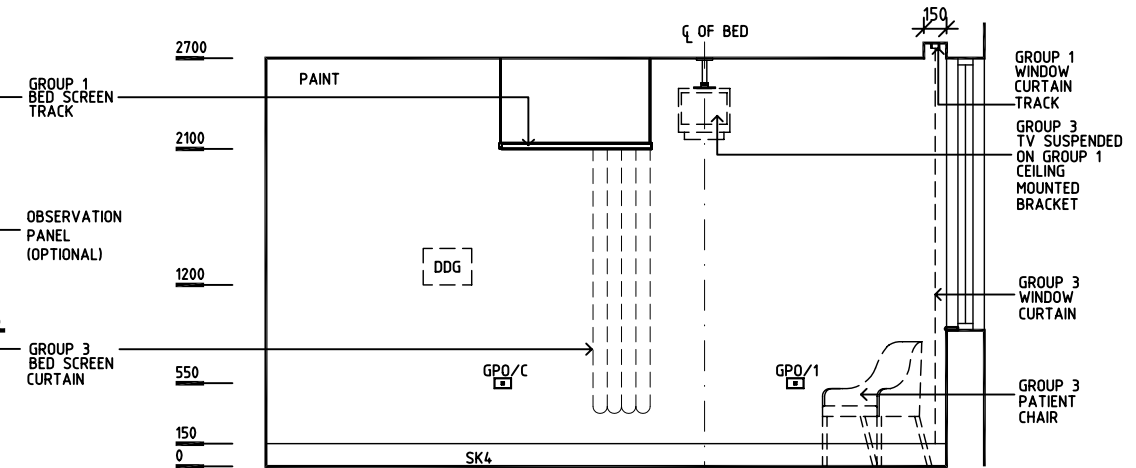
ELEVATION 4
