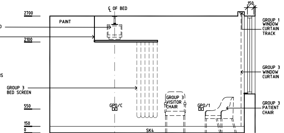
ELEVATION 4
