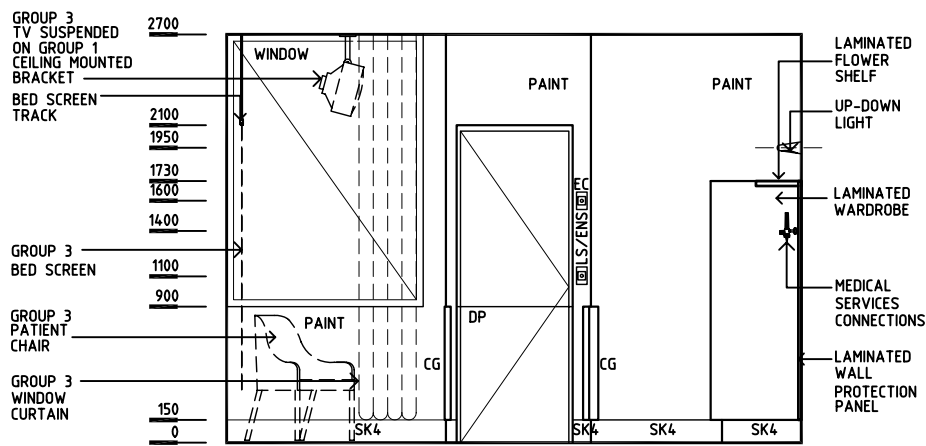
ELEVATION 1
