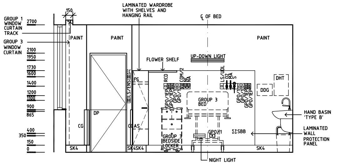
ELEVATION 2
