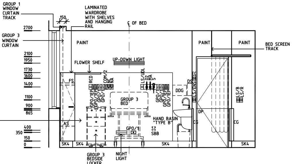
ELEVATION 2
