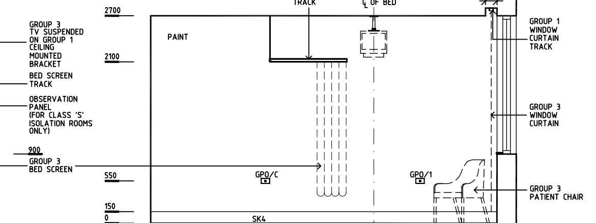
ELEVATION 4
