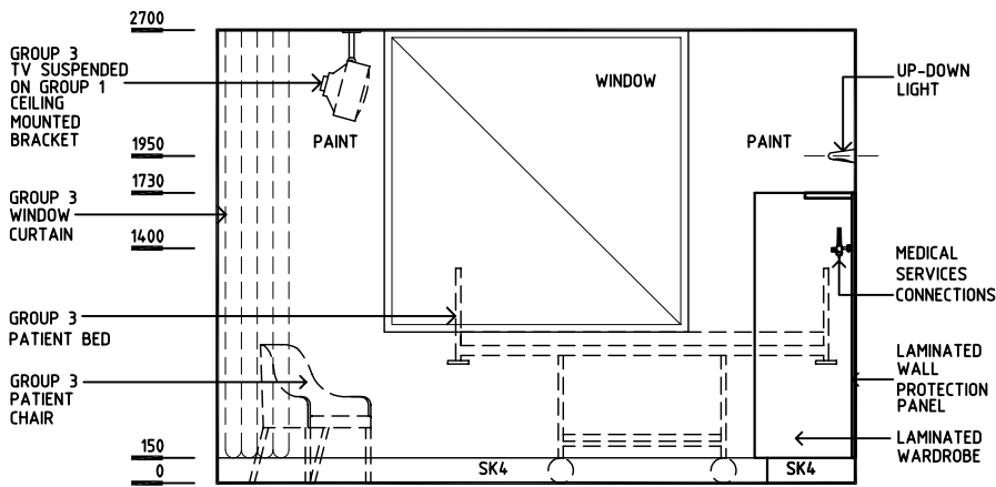
ELEVATION 1
