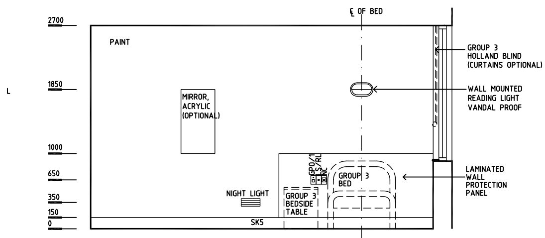
ELEVATION 4
