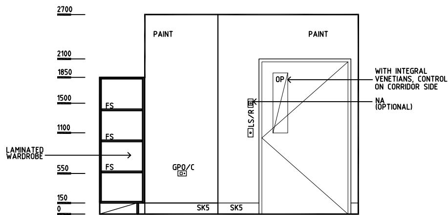
ELEVATION 3
