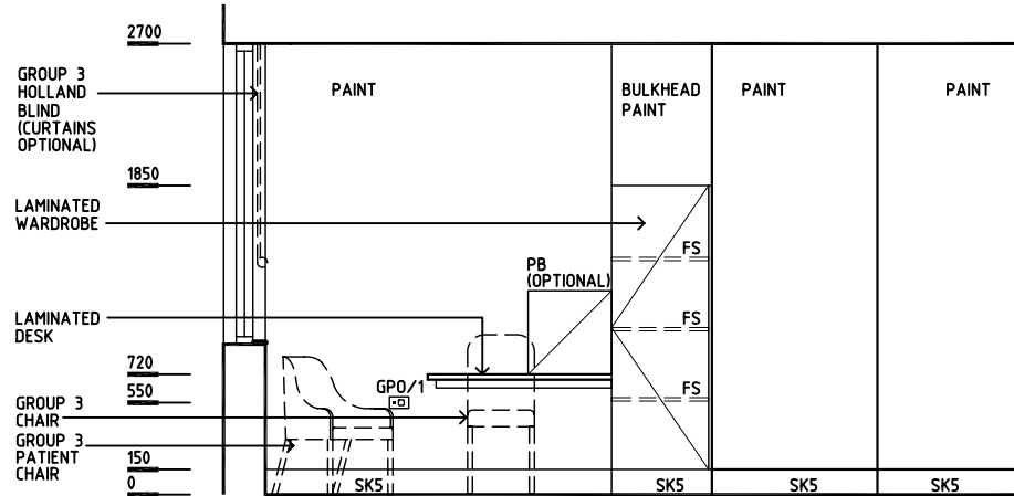
ELEVATION 2
