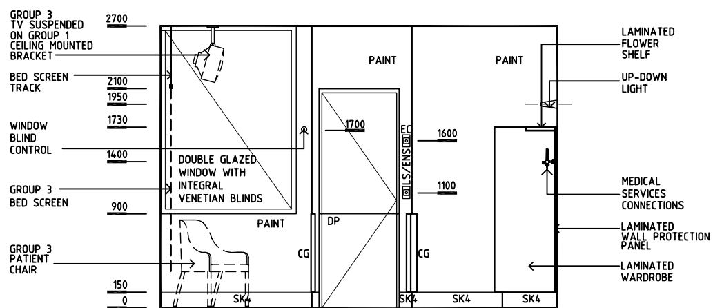
ELEVATION 1
